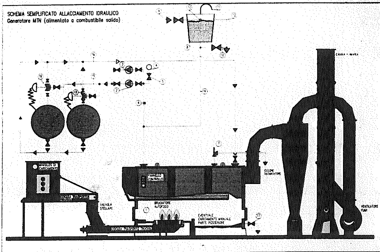
Fig. 1.2 Schema instalației cu cazan de apă caldă MTN 2000 (CT1) / MTN 4000 (CT2), unde: 1. Cazan pentru producerea apei calde; 2. Pompa recirculare; 3. Pompa recirculare (rezerva); 4. Valva cu trei cai; 5. Suport pentru termometrul de control; 6. Suport termometru; 7. Valva descarcare termica (doar pentru manual); 8. Vas de expansiune; 9. Alimentare vas de expansiune; 10. Control de nivel; 11. Conducta de evacuare; 12. Conducta de prea plin; 13. Racord descarcare vas de expansiune; 14. Coducta de siguranta; 15. Conducte de alimentare (tur); 16. Conducte de retur; 17. Conducta evacuare inferioara; 18. Valve de termoreglare; 19. Cos de fum
